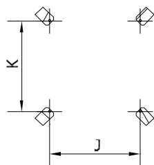
A-A Foot-print ( 1:25 )
