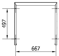
A-A ( 1 : 25 ) Footprint
